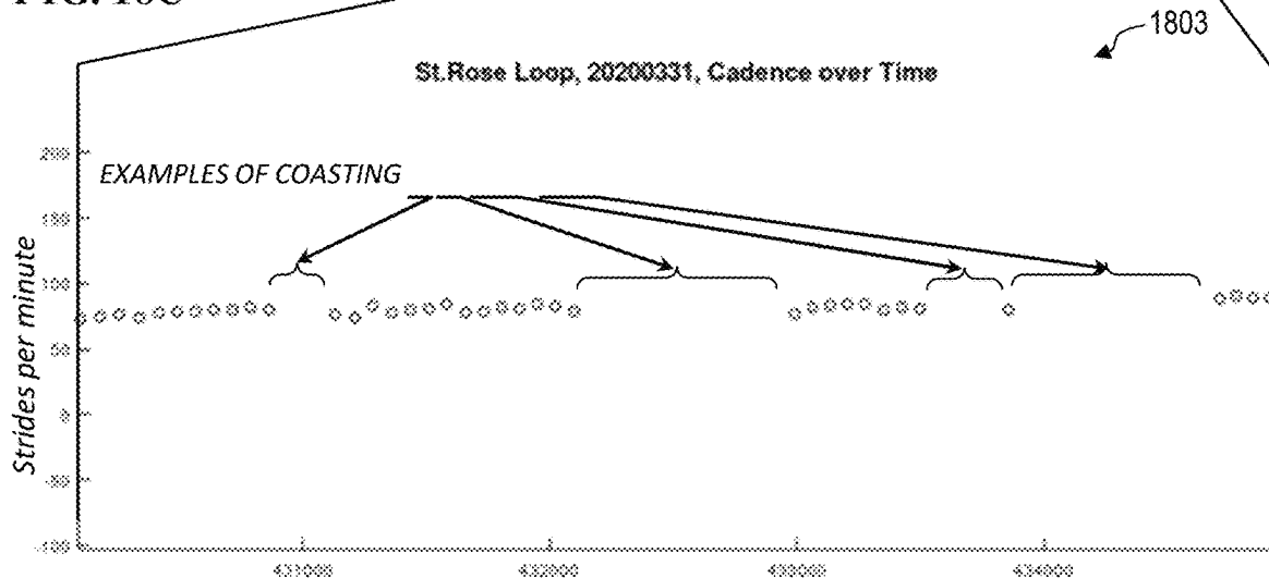
FIG. 18C
